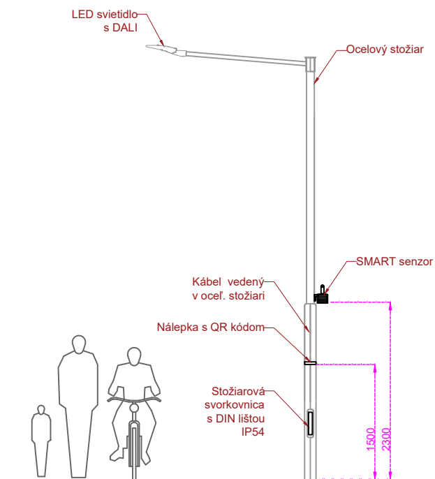
LED svietidlo a SMART senzor s pripojením na LC v stožiarovej svorkovnici
