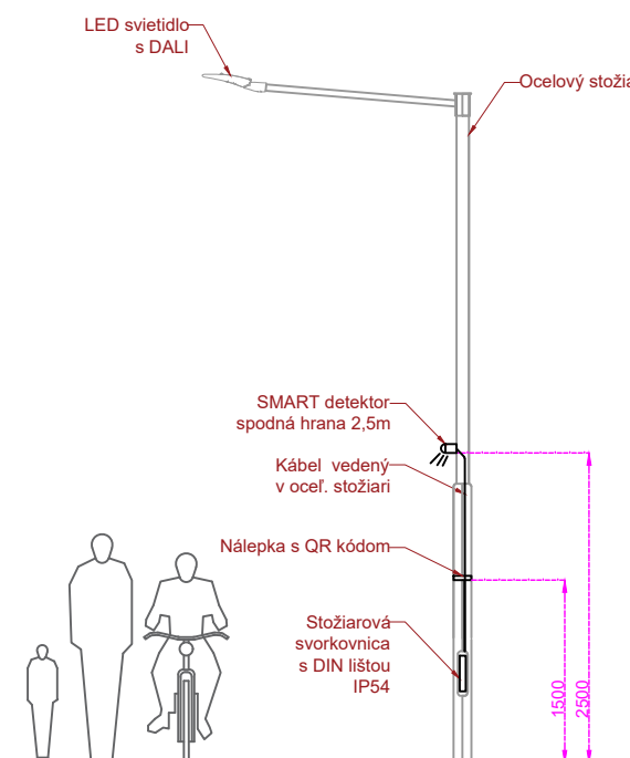
LED svietidlo a SMART detektor s pripojením na LC v stožiarovej svorkovnici
