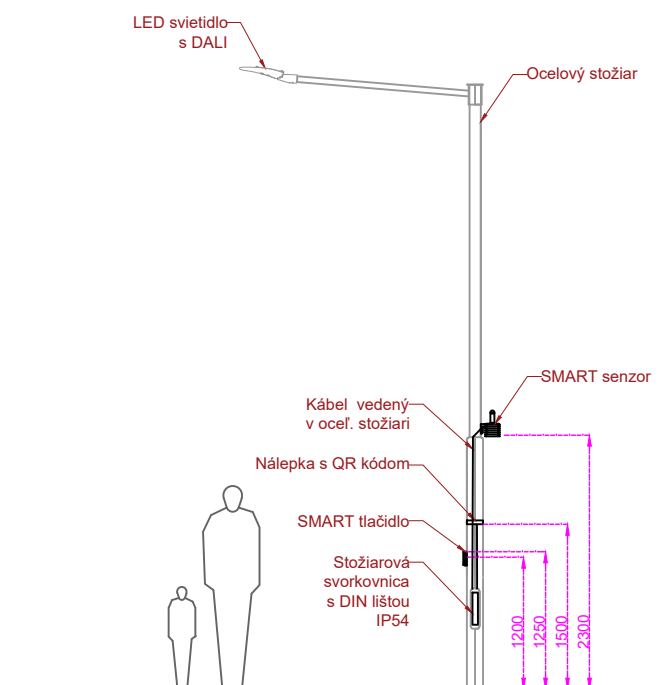
LED svietidlo v kombinácii so SMART senzorom a SMART tlačidlom s pripojením na LC v stožiarovej svorkovnici
