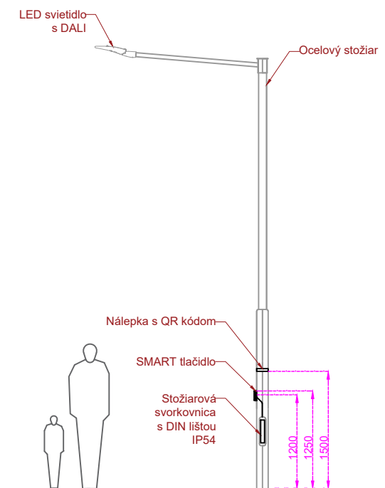
LED svetidlo a SMART tlačidlo s pripojením na LC v stožiarovej svorkovnici
