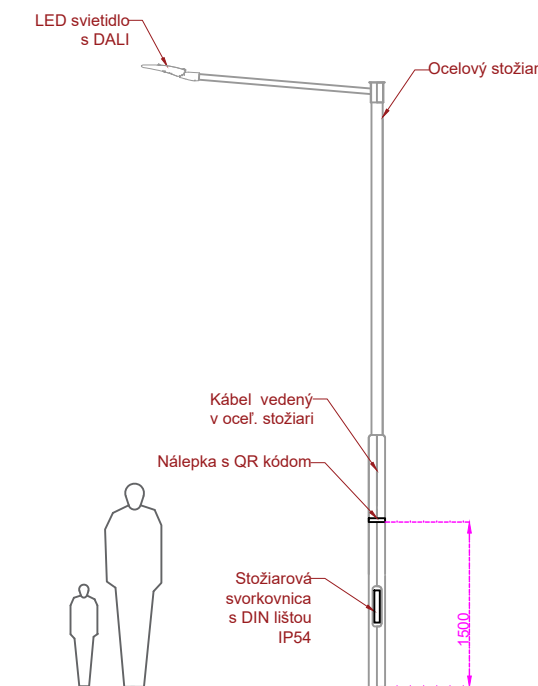
LED svietidlo s pripojením na LC v stožiarovej svorkovnici
