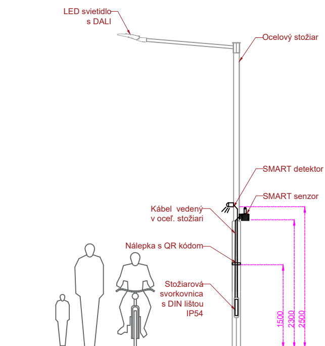
LED svetidlo v kombinácii so SMART senzorom a SMART detektorom s pripojením na LC v stožiarovej svorkovnici
