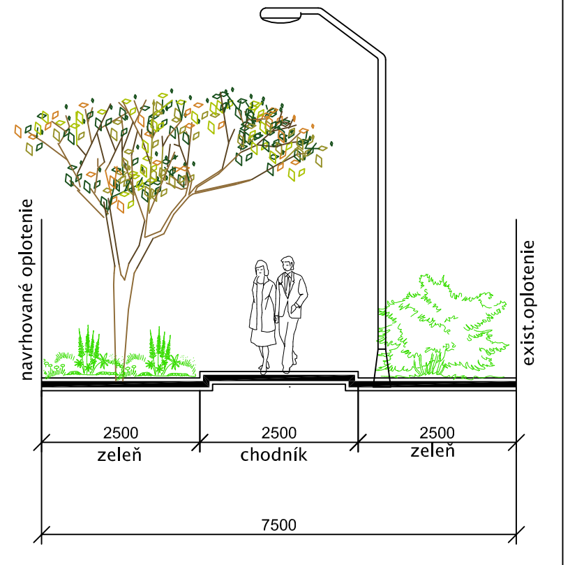
H – uličný profil pre peších – š.4–7,5m
