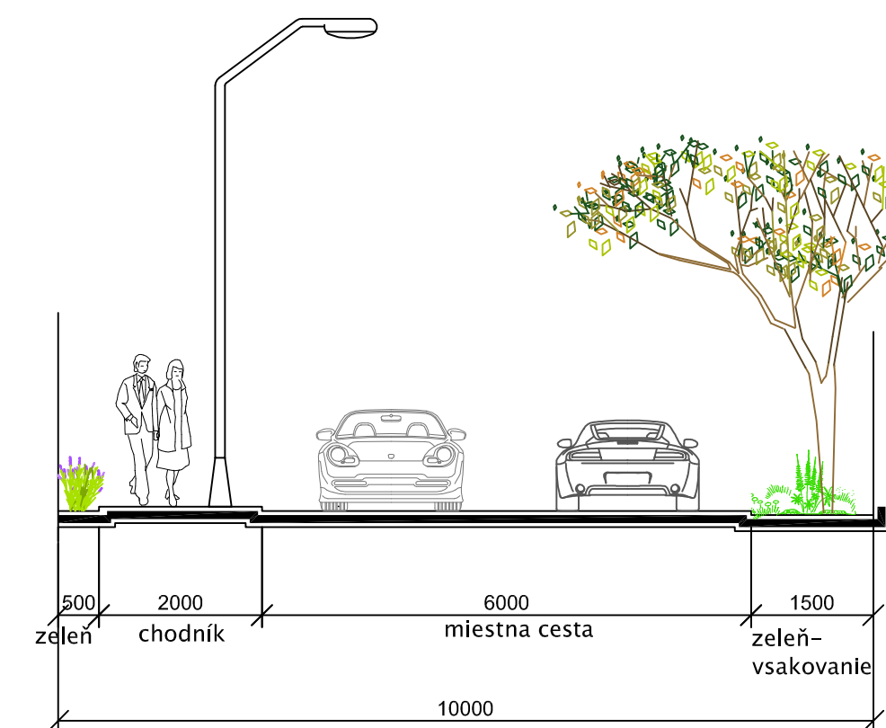
F2 –obytná zóna jednosmerná– š.9,5–10,5m
