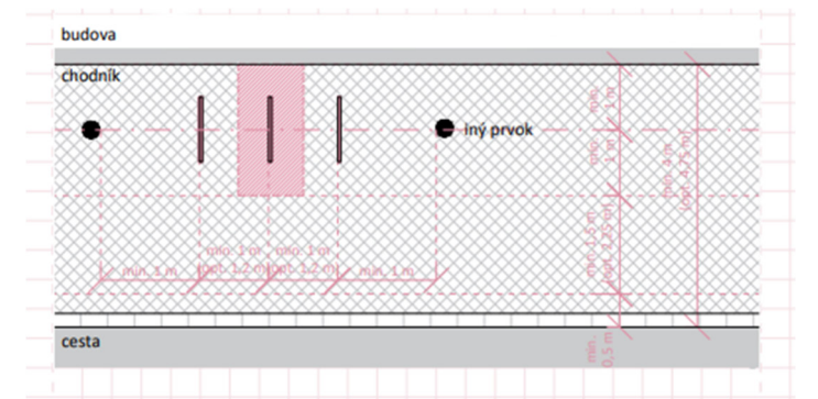
Priečne umiestnenie pri budove
