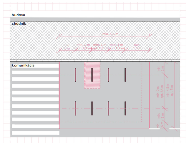
Cyklostanov v dvoch radoch priečne. Hrubá línia označuje použitie ochranných prvkov
