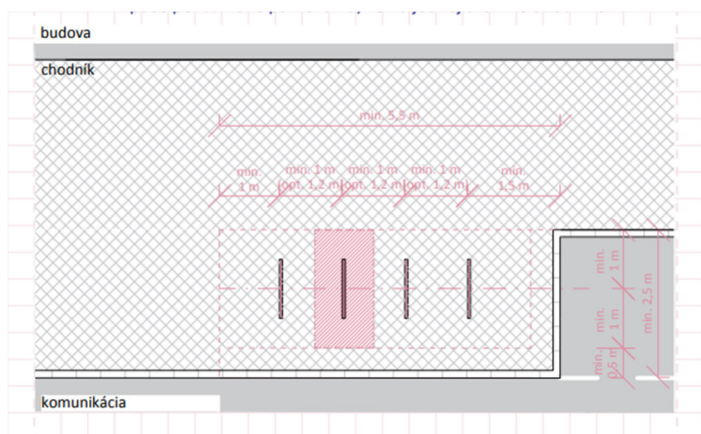
Umiestnenie v páse pozdĺžneho parkovania, na jednej úrovni s chodníkom
