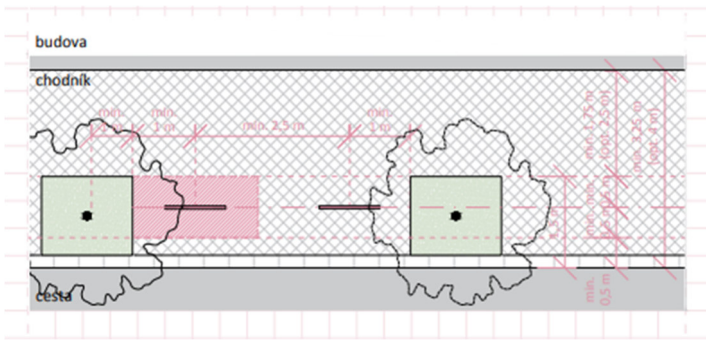
Pozdĺžne umiestnenie v stromoradi
