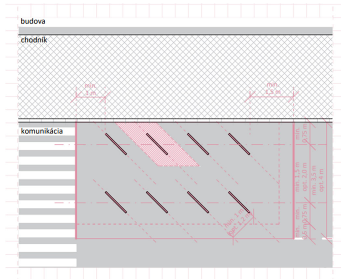
Cyklostojany v dvoch radoch šikmo. Hrubá línia označuje použitie ošranných prvkov
